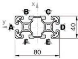
40x80L Strut
