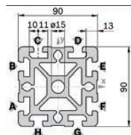
90x90 Strut
