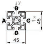
45x45 Strut
