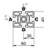
45x60 Strut
