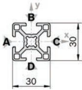
30x30 Strut
