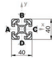
40x40L Strut
