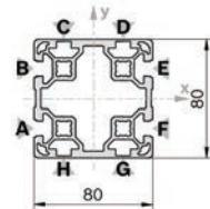
80x80L Strut
