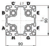
90x90L Strut
