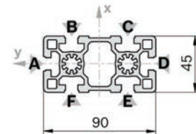
45x90 Strut
