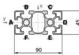
45x90L Strut
