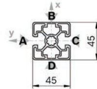
45x45L Strut
