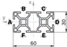
30x60 Strut
